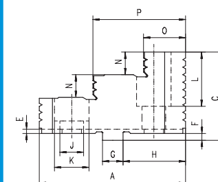
Ø 10"-32"
